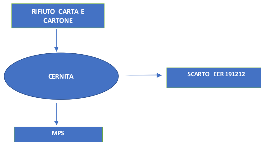
Figura 4: diagramma a blocchi trattamento carta e cartone - step 2c
