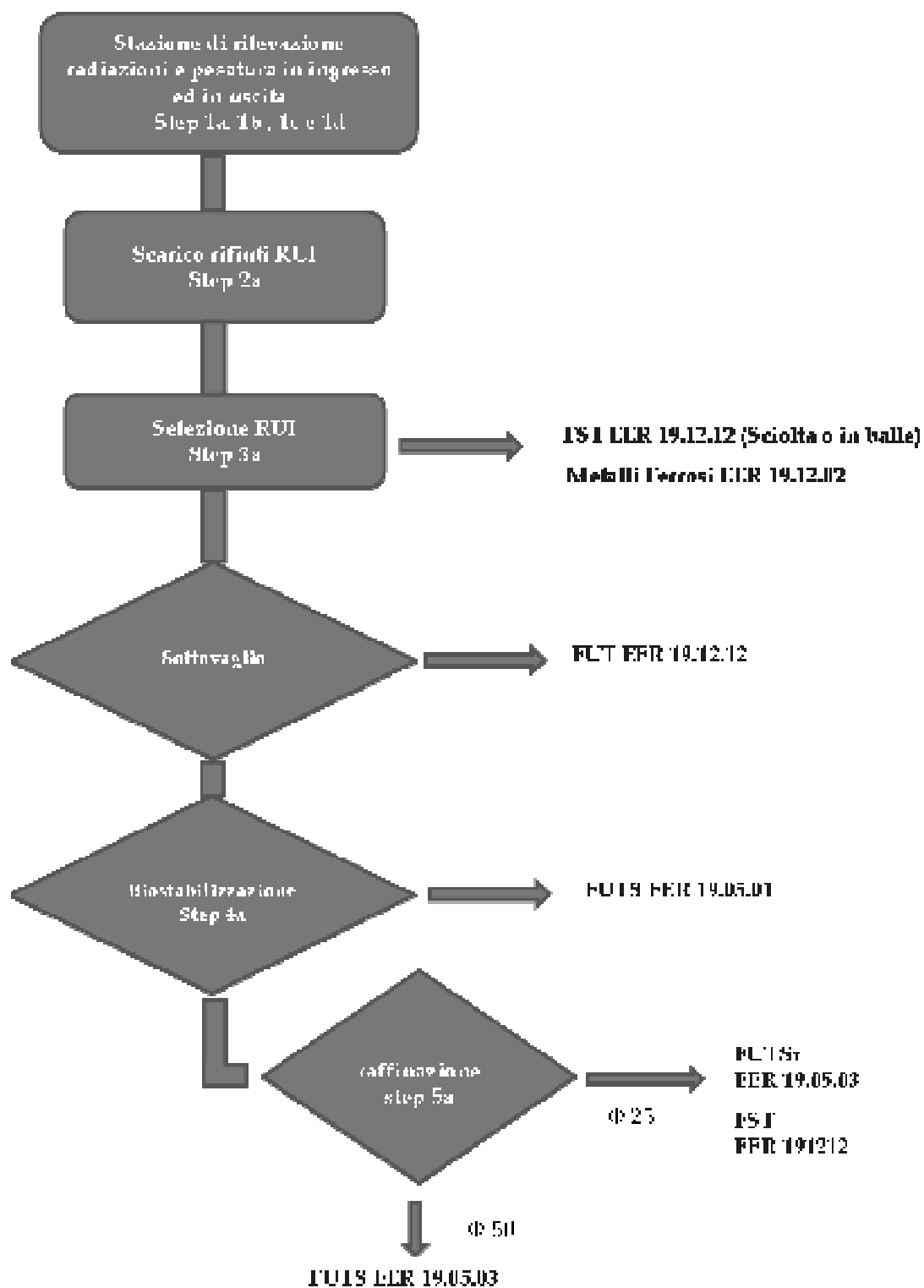
Figura 2: diagramma a blocchi TMB
