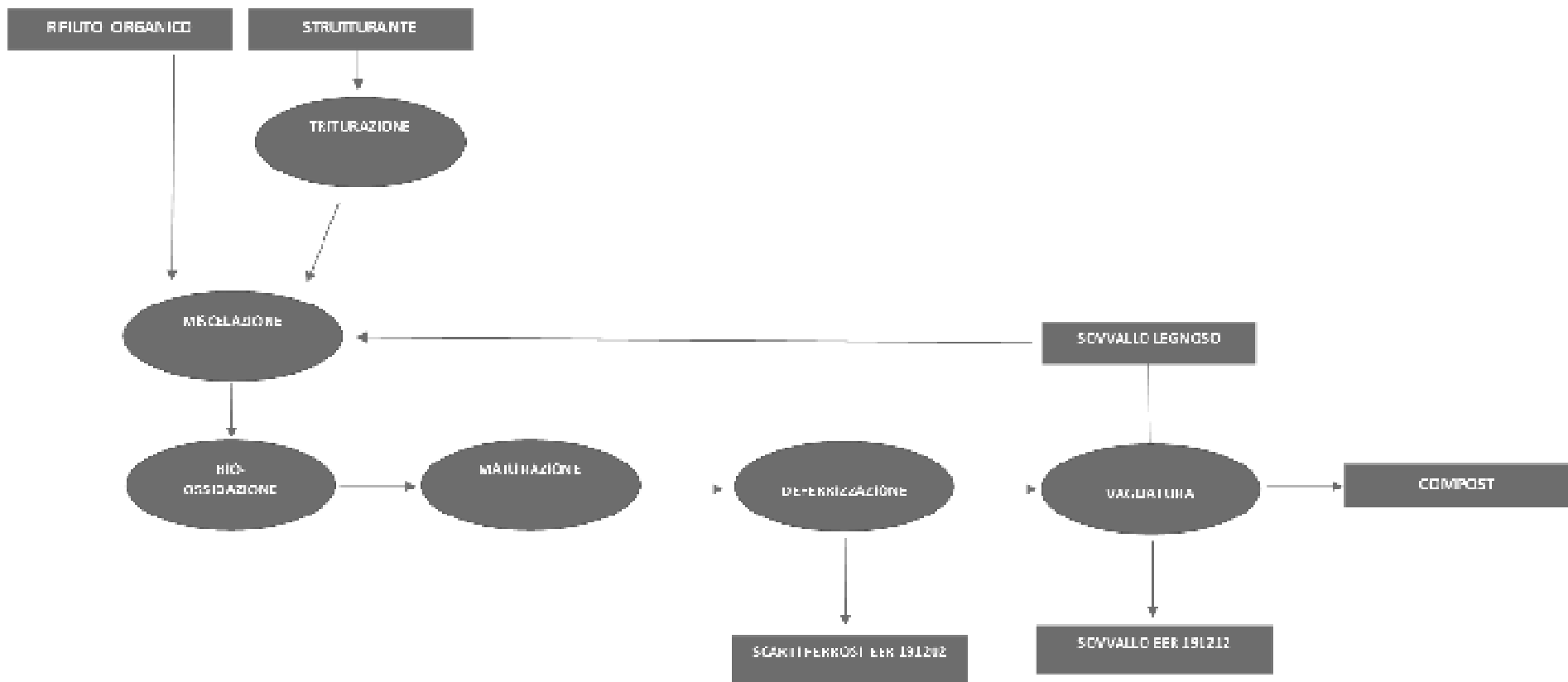
Figura 6: diagramma a blocchi compostaggio - Step 2d
